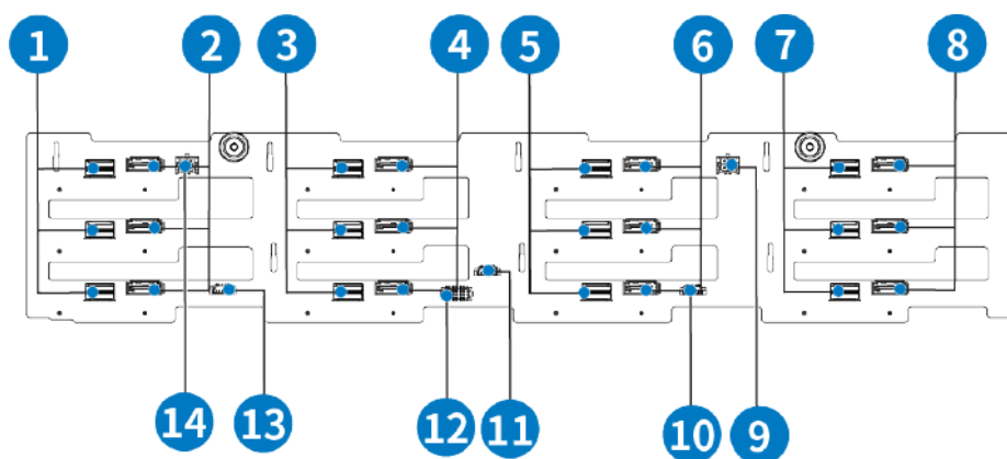
Рисунок 6 – Бэплейн (кроссплата) Тринити (на 12 накопителей). Вид сзади
