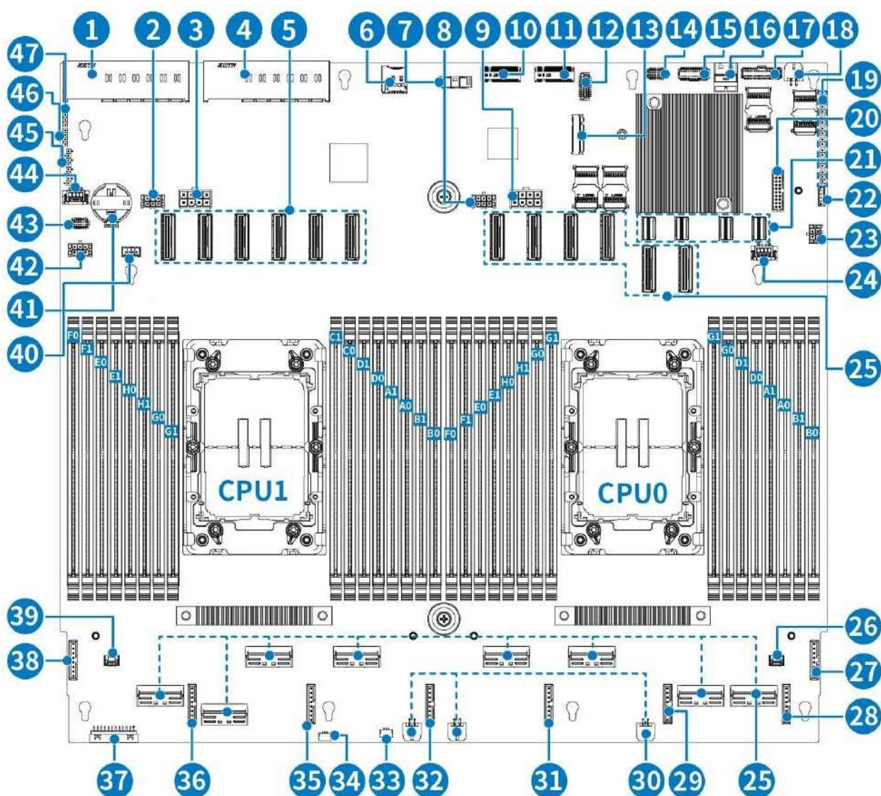
Рисунок 1 – Внешний вид материнской платы Тринити
