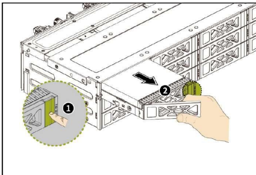
Рисунок 29 – Извлечение накопителя
