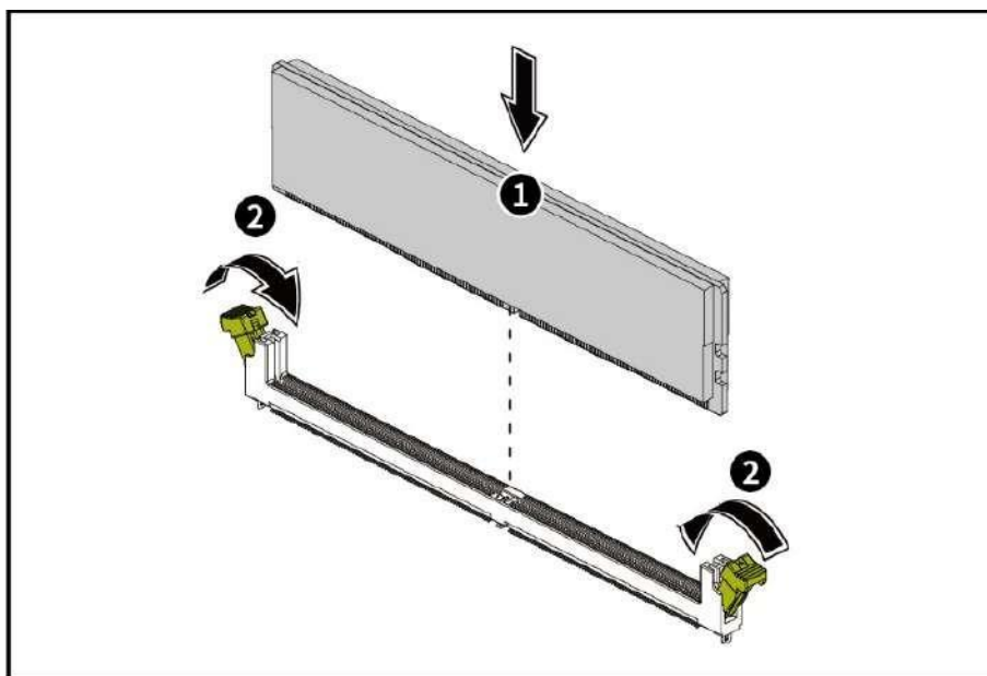
Рисунок 70 – Установка памяти
