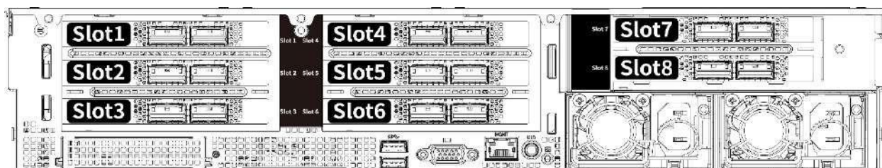
Рисунок 18 – Расположение слотов PCIe (8 шт.)
