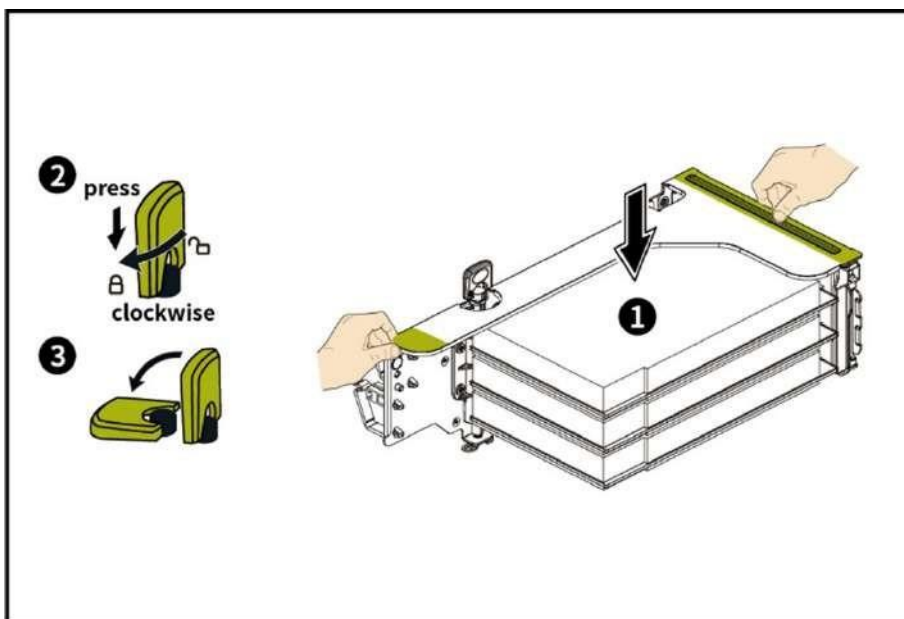
Рисунок 46 – Установка модуля 3PCIe
