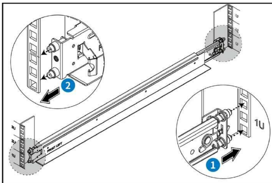
Рисунок 20 – Установка направляющих
