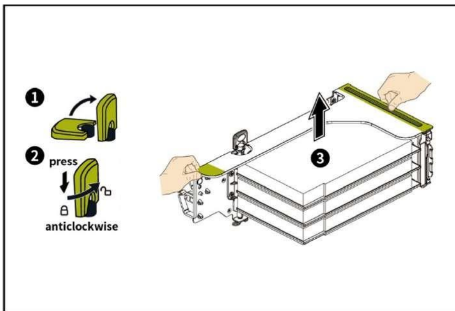
Рисунок 45 – Демонтаж модуля 3PCIe
