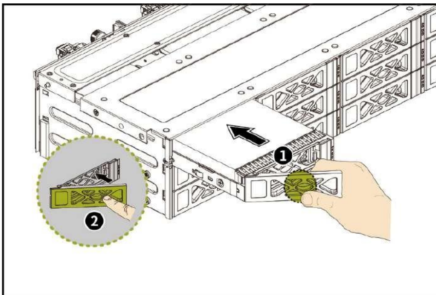
Рисунок 30 – Установка накопителя
