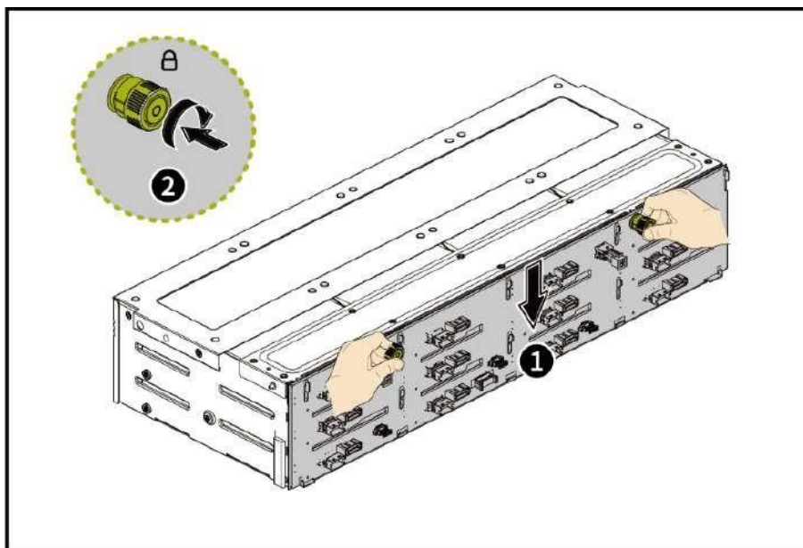
Рисунок 42 – Установка бэкплейна
