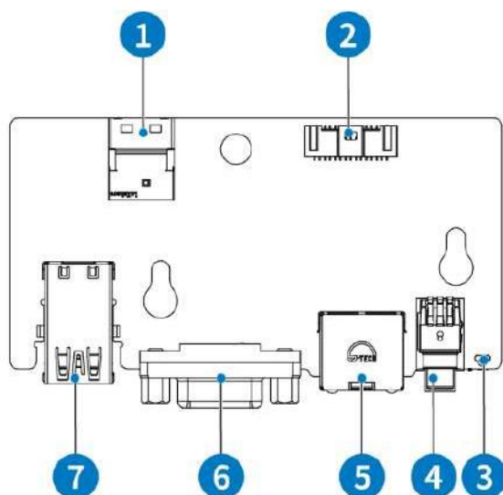
Рисунок 11 – Внешний вид платы IOM
