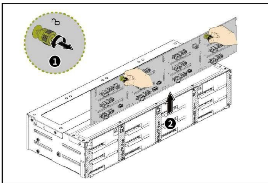
Рисунок 41 – Снятие бэкплейна
