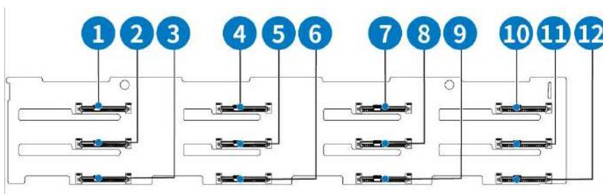
Рисунок 5 – Бэплейн (кроссплата) Тринити (на 12 накопителей). Вид спереди
