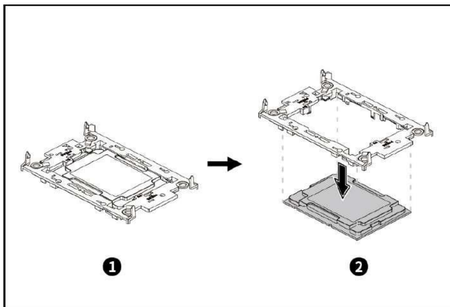
Рисунок 63 – Извлечение процессора из кронштейна
