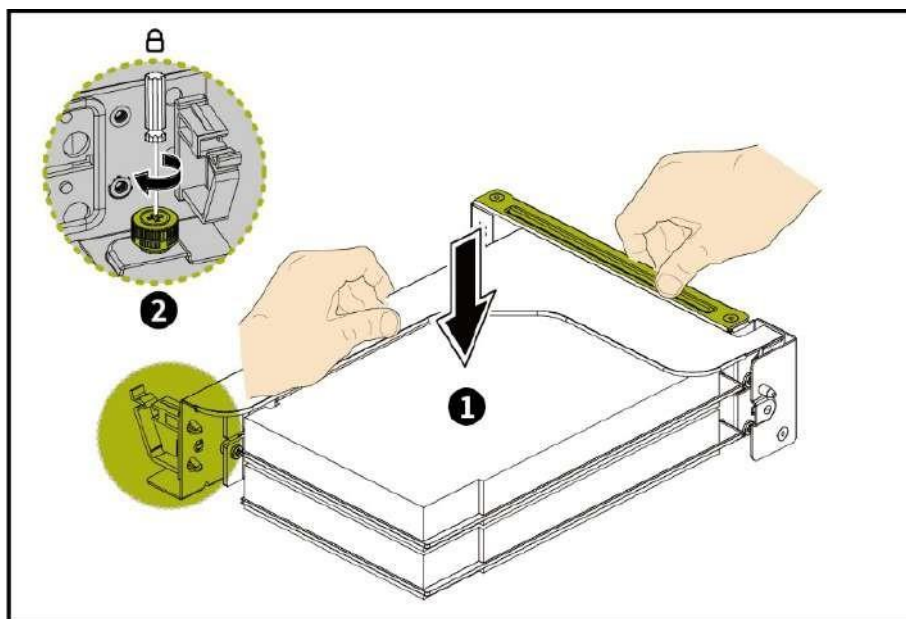
Рисунок 48 – Установка модулей 2PCIe
