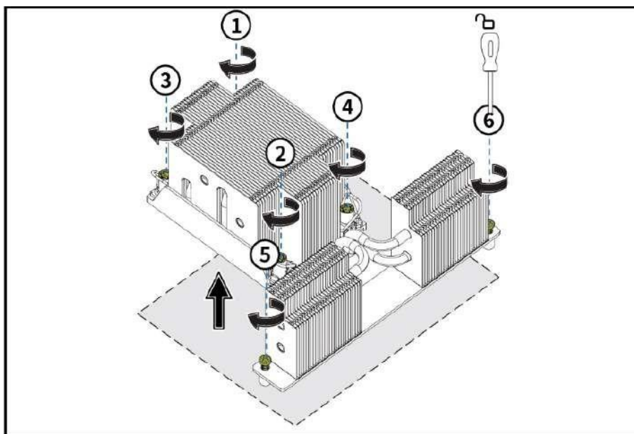
Рисунок 59 – Демонтаж радиатора
