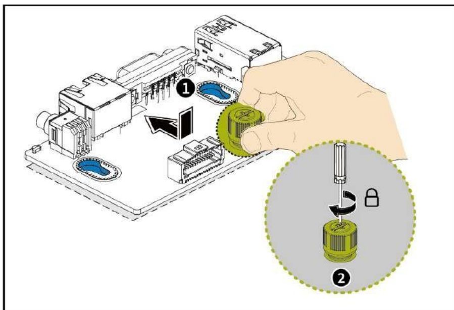
Рисунок 58 – Установка платы IOM
