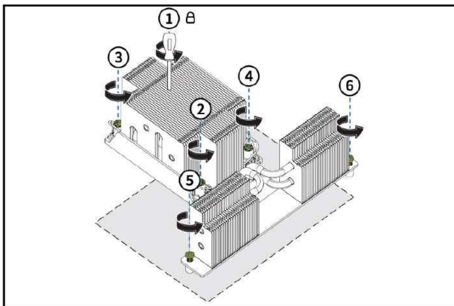
Рисунок 60 – Установка радиатора
