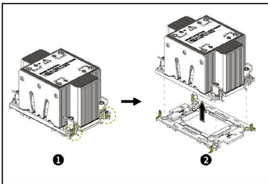
Рисунок 62 – Отделение радиатора от процессора с кронштейном
