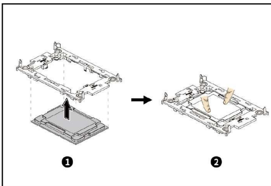
Рисунок 66 – Установка процессора в кронштейн
