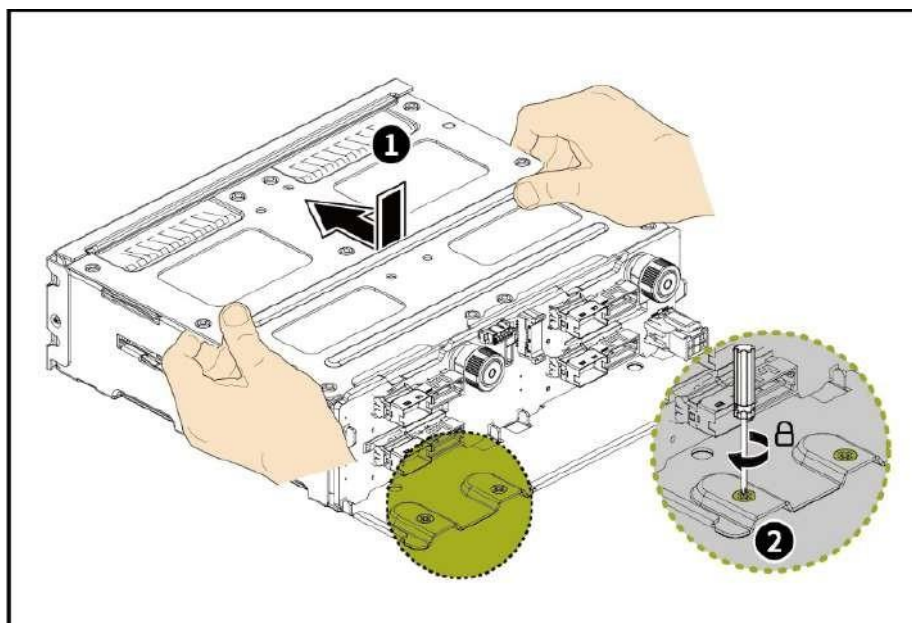
Рисунок 44 – Установка заднего отсека накопителей
