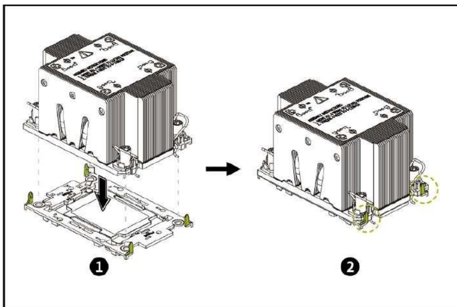
Рисунок 67 – Установка радиатора
