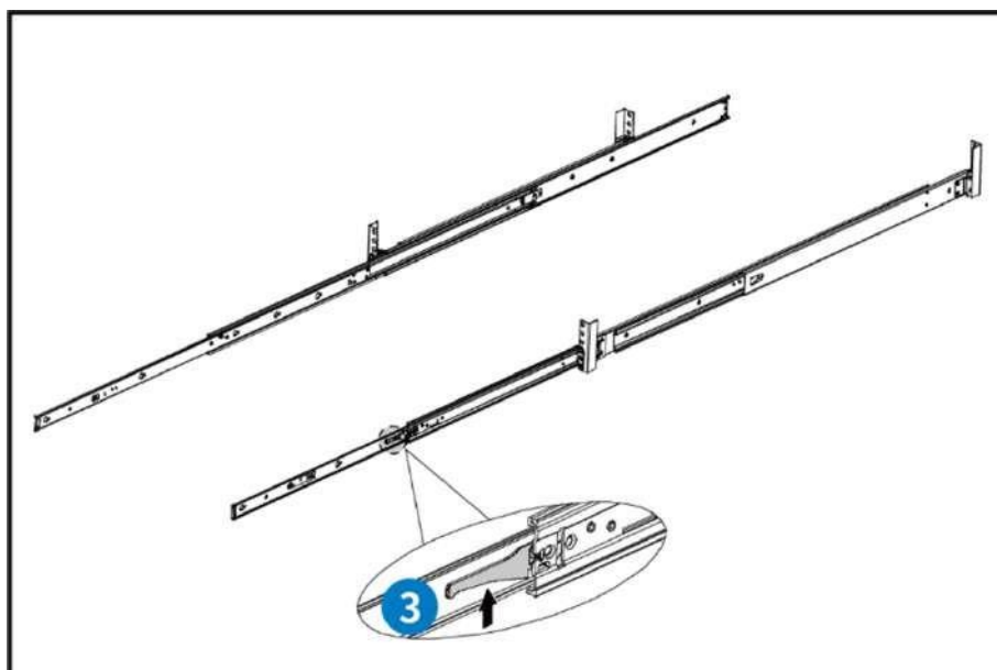
Рисунок 23 – Установка направляющих
